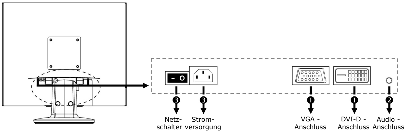
(Abb.: Rückseite Bildschirm)
