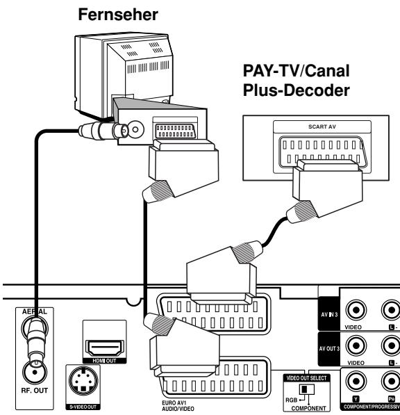
Rückseite des Recorders
