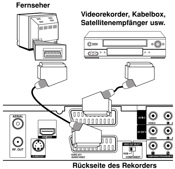
Rückseite des Recorders
