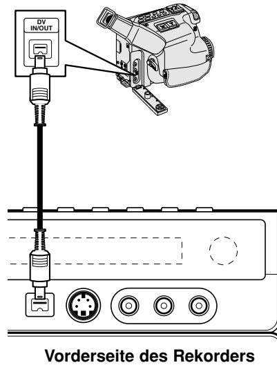
Vorderseite des Rekorders
